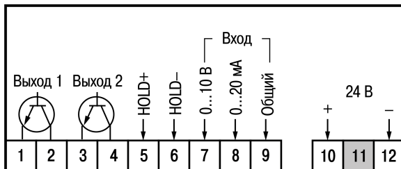
Рисунок 5.1 – Назначение контактов клеммника
