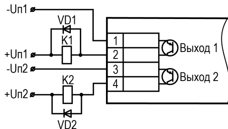
Рисунок 5.3 – Схема подключения реле к прибору
