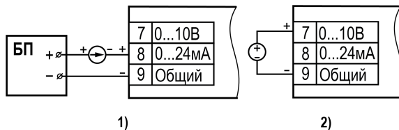
Рисунок 5.2 – Схема подключения к прибору: 1) датчиков с выходными сигналами постоянного тока 0...5 мА, 0...20 мА и 4...20 мА, 2) датчиков с выходными сигналами постоянного напряжения 0...1 В и 0...10 В
